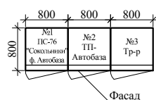
План расположения камер в РУ М 1:100
